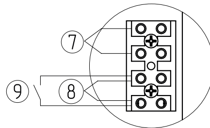
Подключение датчиков
