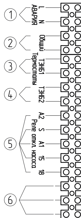
Внешние подключения
