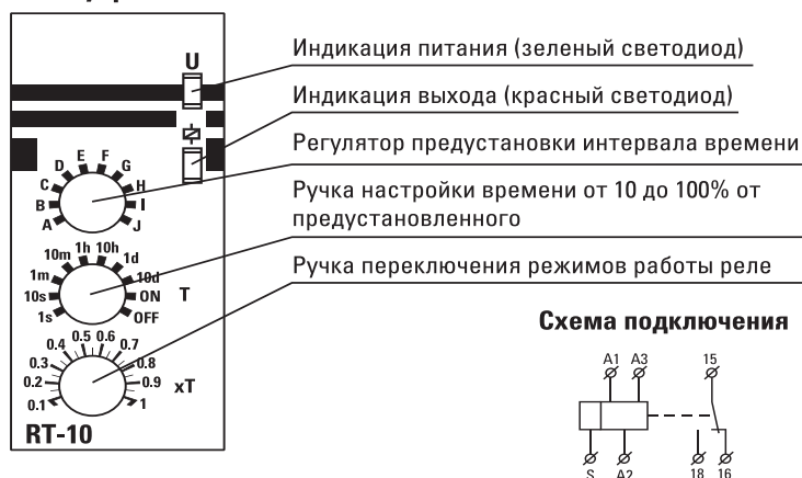
Рис.7 Панель управления реле
