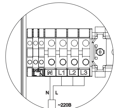
Подключение 220 В
