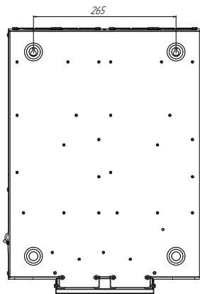
Рисунок 23. Задняя панель стабилизаторов IS8000 и IS10000
