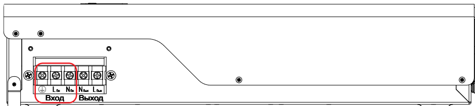
Рисунок 27. Стабилизатор Штиль IS7000. Выводы «Вход \perp -L-N»
