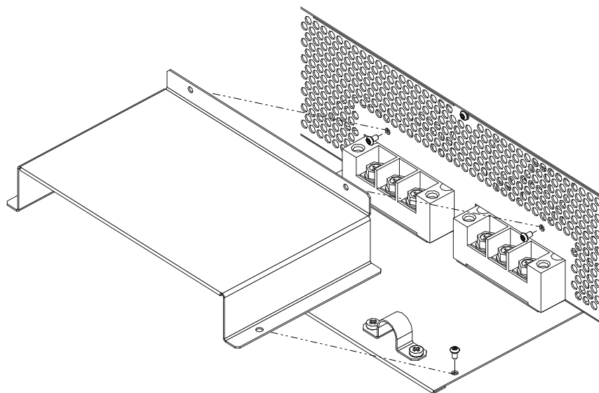
Рисунок 35. Крепление защитного кожуха у стабилизаторов Штиль IS8000 и IS10000
