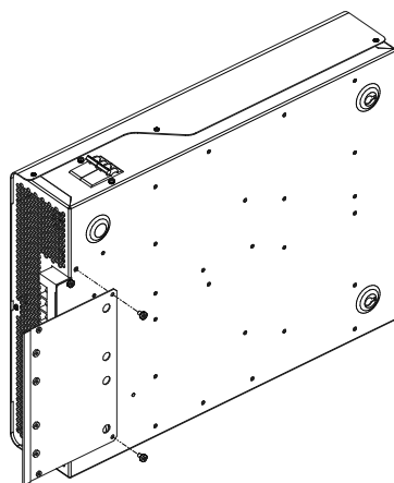
Рисунок 22. Задняя панель стабилизатора IS7000
