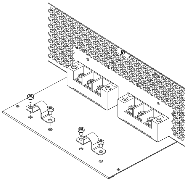
Рисунок 34. Соединение скобы фиксации кабелей с пластиной фиксации защитного кожуха у стабилизаторов Штиль IS8000 и IS10000
