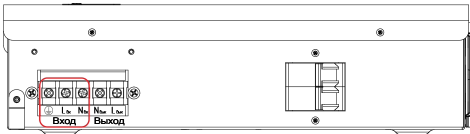
Рисунок 26. Стабилизатор Штиль IS5000. Выводы «Вход \perp -L-N»
