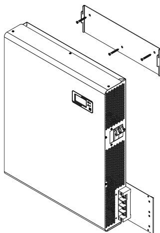
Рисунок 13. Крепление стабилизатора IS12000 (крепление стабилизатора IS15000 аналогично)
