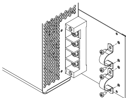
Рисунок 22. Соединение скобы фиксации кабелей с пластиной фиксации защитного кожуха у стабилизаторов IS12000 и IS15000
