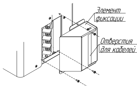
Рисунок 24. Крепление защитного кожуха у стабилизатора IS20000
