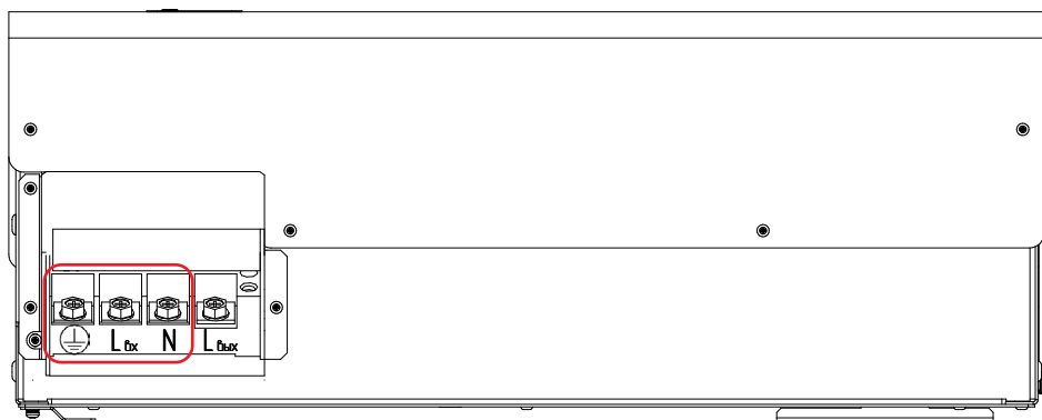
Рисунок 19. Стабилизатор ШТИЛЬ IS20000. Выводы «⏏-Lвх-N».
