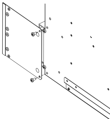
Рисунок 13. Крепление стабилизатора IS12000 (крепление стабилизатора IS15000 аналогично)
